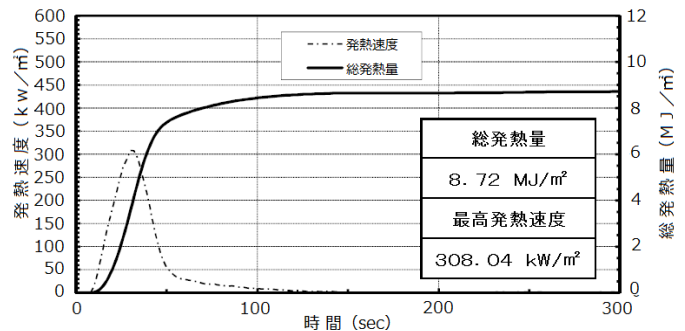
【図1】接着剤5gの発熱総量及び総発熱速度(試験体 A14)
