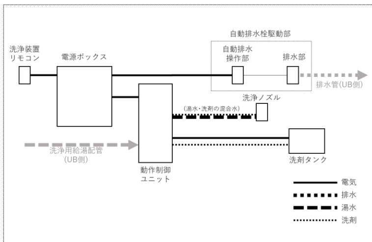
図-1 自動浴槽洗浄システムの例
