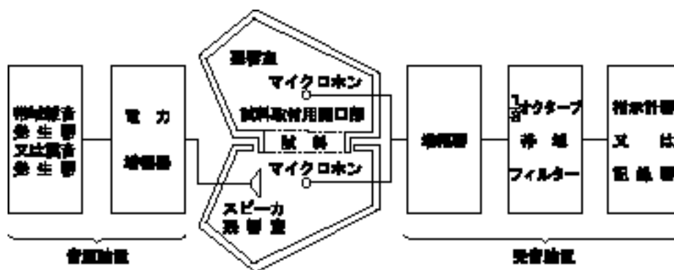
図9-1 試験装置
