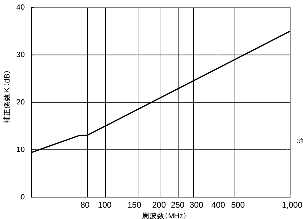
図2 補正係数
