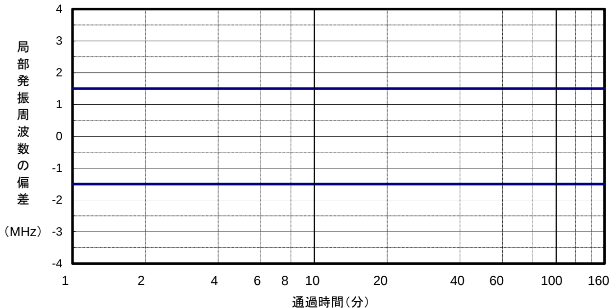
温度安定度
