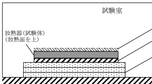
放熱器(試験体)の支持方法
