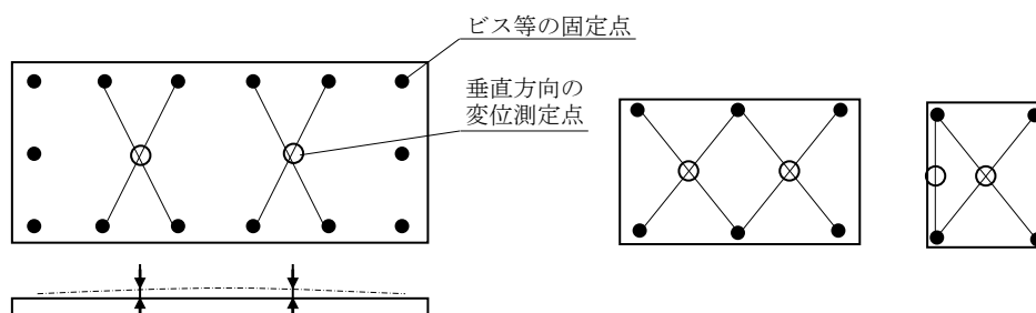
放熱器(試験体)の垂直方向の変位測定箇所(例)
