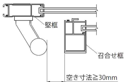
図-15 把手と召合わせ框との空き寸法
