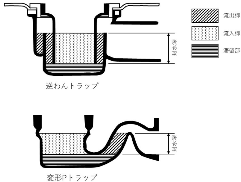
図-3 トラップの各部位の名称
