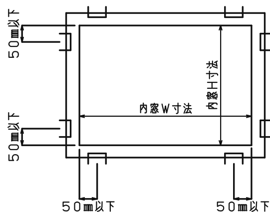
図-2 取付けステープルの内部縁端からの距離
