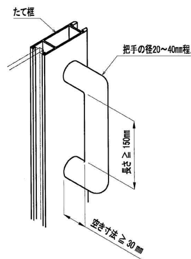
図-12 把手の寸法
