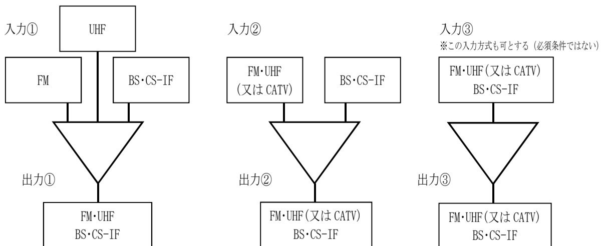
図-2 ブロック図（SH-1）
