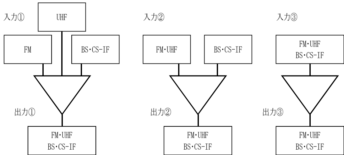
図-3 ブロック図 (SH-UF-1)
