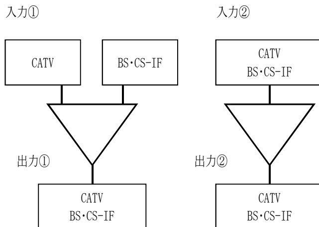
図-4 ブロック図 (CATV-SH-1/SH-P1)
