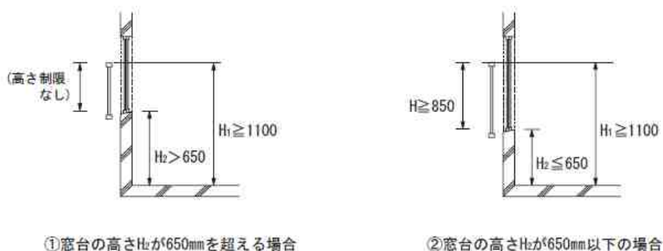
図一窓台の高さによる窓用手すりユニット高さ H の例示
