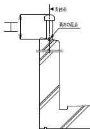
トップレール壁支持 (芯納まり) 図-5
