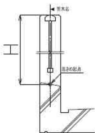
手すり壁支持 (芯納まり) 図-4
