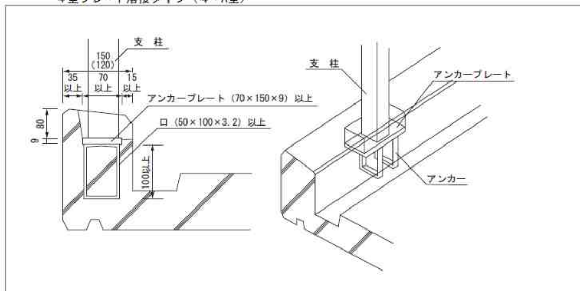
4型プレート溶接タイプ (4-B型)
