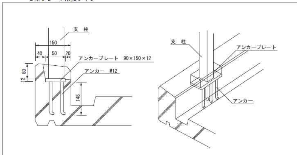
4型プレート溶接タイプ (4-A型)
