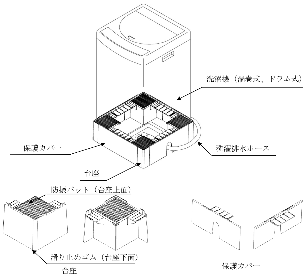
図-1 構成図
