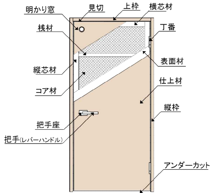
図一5 開戸（フラッシュ戸）の例
