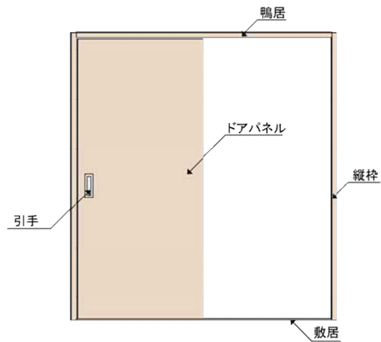
図—7 引戸の例
