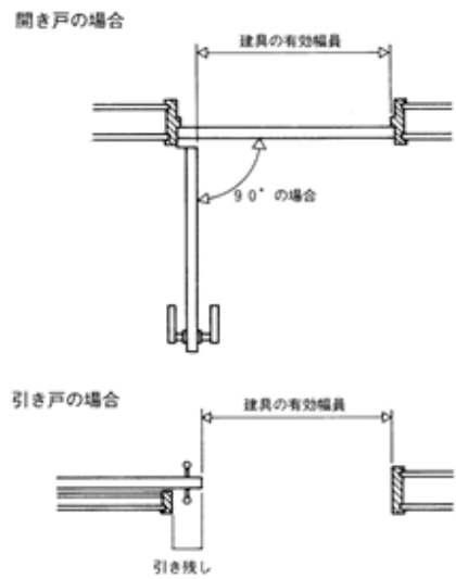
図－１ 玄関ドアの有効幅員
