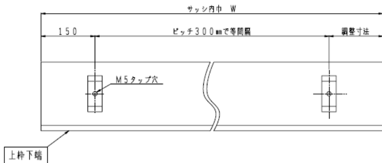
図-3 ドア・クローザの上枠のハンガーレール取付け用タップ加工位置 単位 (mm)
