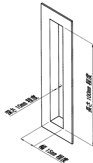
図-8 彫り込み引手寸法の押さえ方
