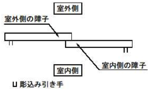
図-6 引違い（出入口以外）の彫込み引手取り付け例
