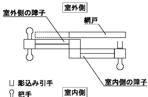
図-9 網戸が有効に機能する例
