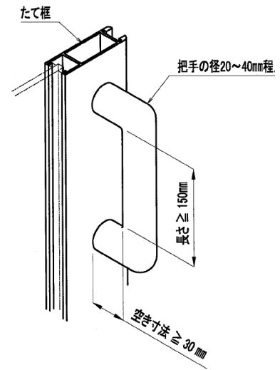
図-11 把手の寸法
