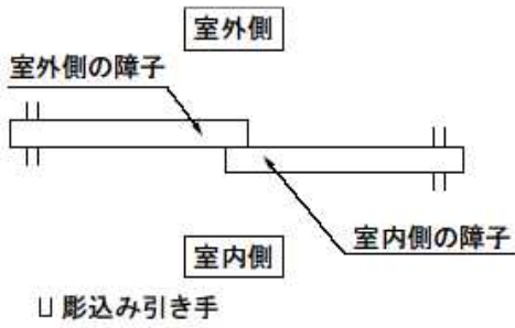
図-5 引違い（出入口）の彫込み引手取り付け例
