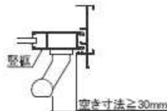
図-13 把手と枠との空き寸法
