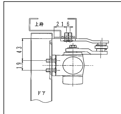
図-4 (開き戸用ドア・クローザ)
