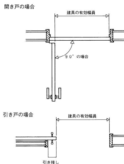
図－1 玄関ドアの有効幅員
