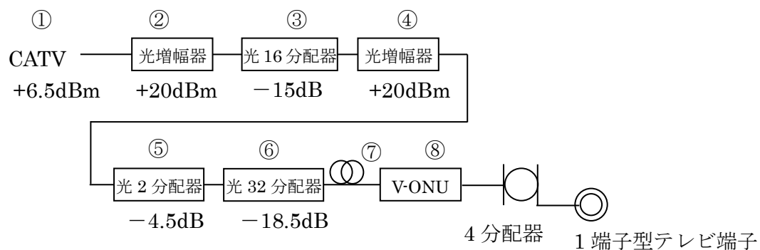
図－１８ 1024 端末(光増幅器 2 段)
