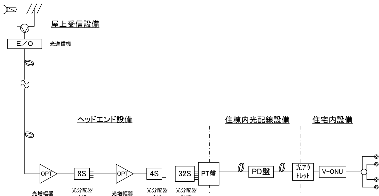
図－7 SMATV システム構成例
