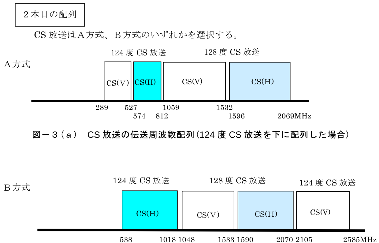
図－3 (b) CS 放送の伝送周波数配列(124 度 CS 放送を上下に配列した場合)
