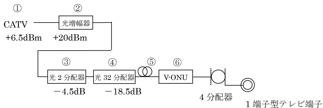
図－１７ 64 端末(光増幅器 1 段)
