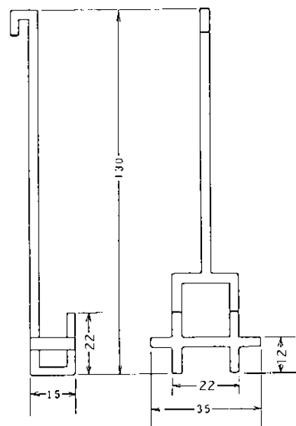
図－9 試験片ホルダー（ガラス製）
