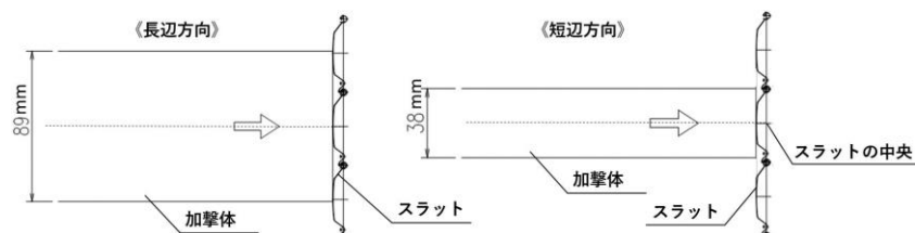
図2 加撃体の向き
