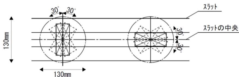
図3 加撃体の許容回転角度
