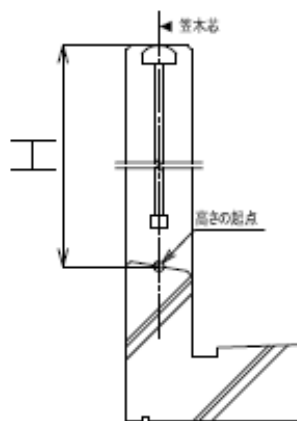
手すり壁支持 (芯納まり)
