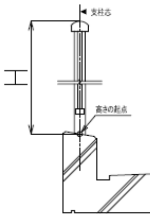
手すり床支持 (芯納まり)
