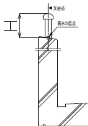
トップレール腰壁支持 (芯納まり)
