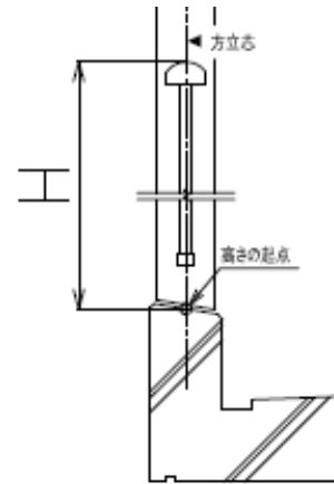
手すり方立て支持 (芯納まり)
