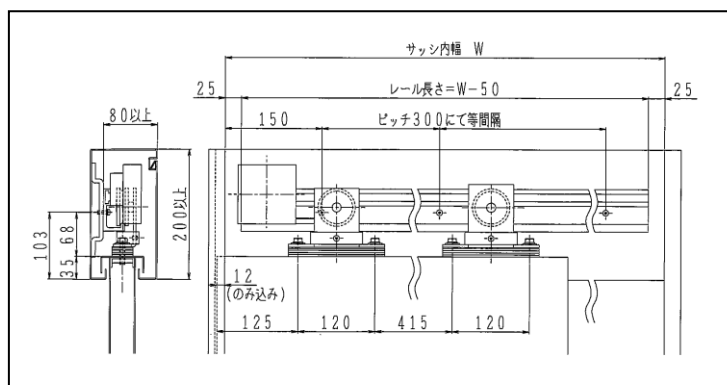
図-5 (引き戸用ドア・クローザ)
