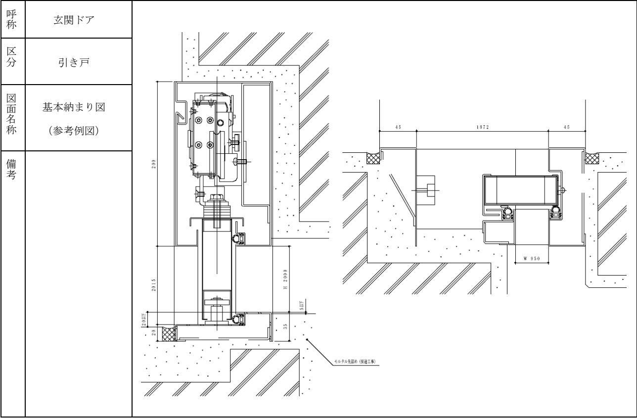
i) 引き戸基本納まり図
