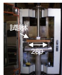
写真1 温度調整炉付き圧縮試験機
