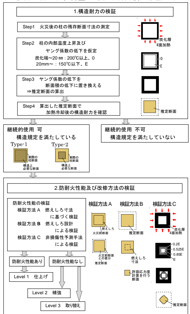
図7 柱の火災診断及び改修フローチャート
