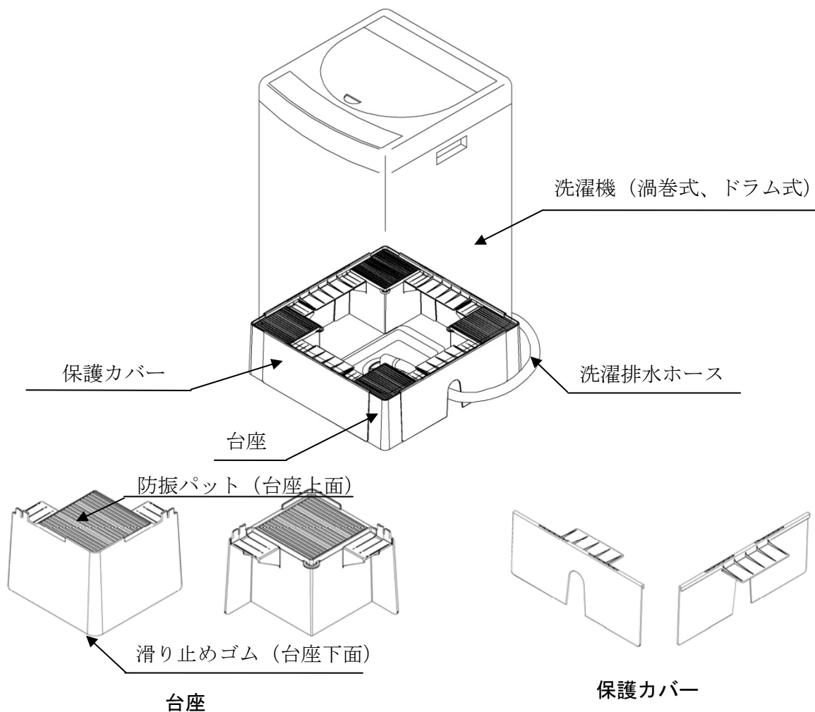
図-1 構成図
