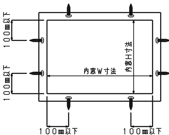
図-1 取付けねじの内部縁端からの距離
