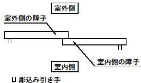
図-6 引違い（出入口以外）の彫込み引手取付け例
