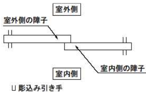
図-5 引違い（出入口）の彫込み引手取付け例
