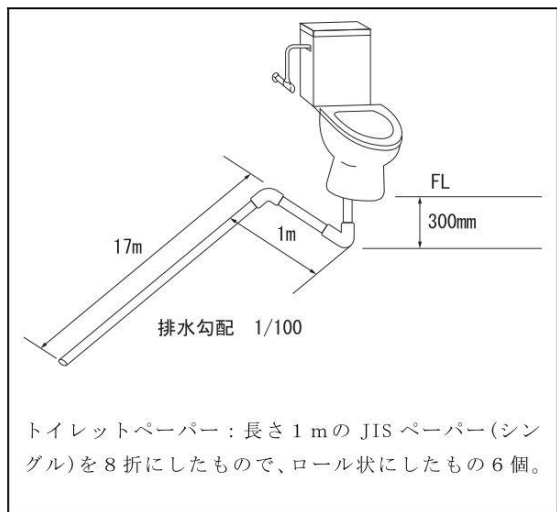
試験方法改正案（搬送性能：B L -bs）
