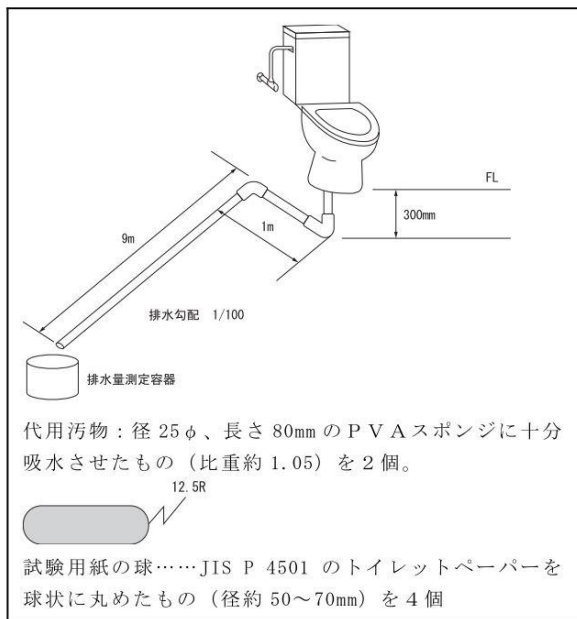
性能試験方法（搬送性能：一般型）
