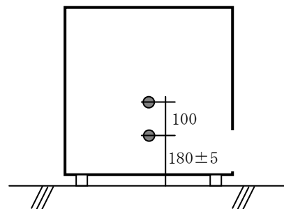
別図 2-4 据置形の追いだき機能付給湯器（浴室内設置型を除く）の配管接続位置
