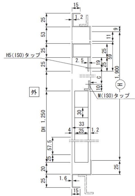
A-A矢視図
