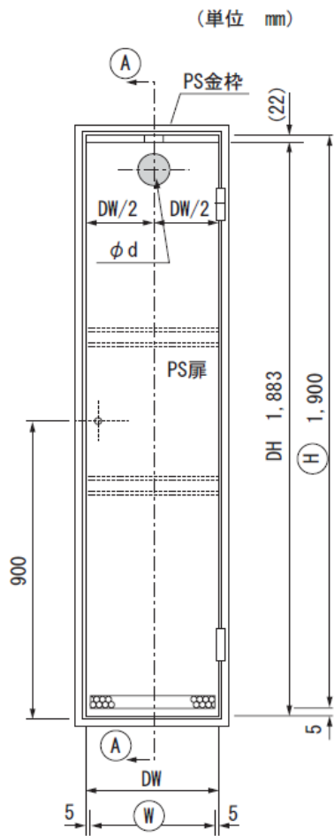
給湯器取付けボックスの取付け部寸法
