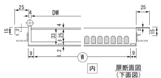
別図 1-1 パイプシャフト設置形(直付型)の取付金枠図
