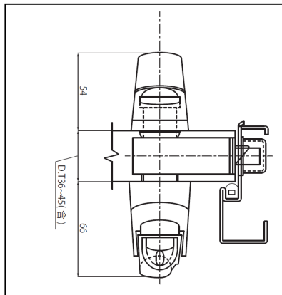
図-3（プッシュプルハンドル錠）対象外
