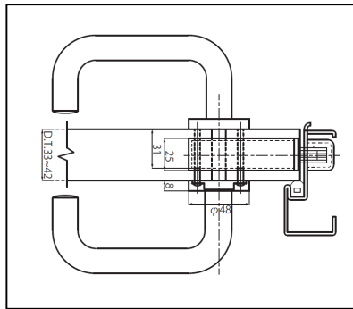
図-1（レバーハンドル錠）
