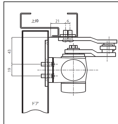
図-4（開き戸用ドア・クローザ）
